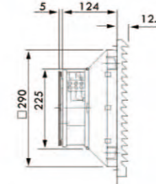
风机过滤器 FK6626.230
