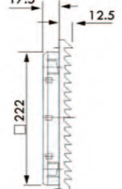
出口过滤器 FK6625.300
