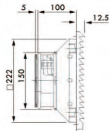
风机过滤器 FK6625.230
