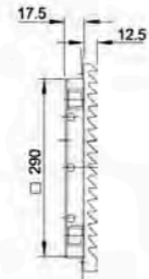
出口过滤器 FK6626-D.300
