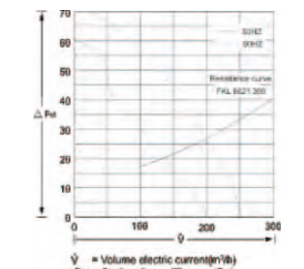
功率特性曲线
