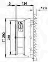
风机过滤器 FK6626-D.230
