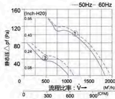
功率特性曲线
